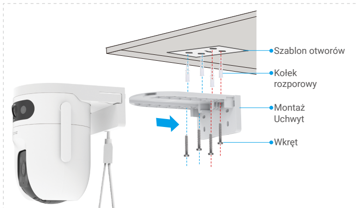
Rys. 1 Montaż sufitowy
