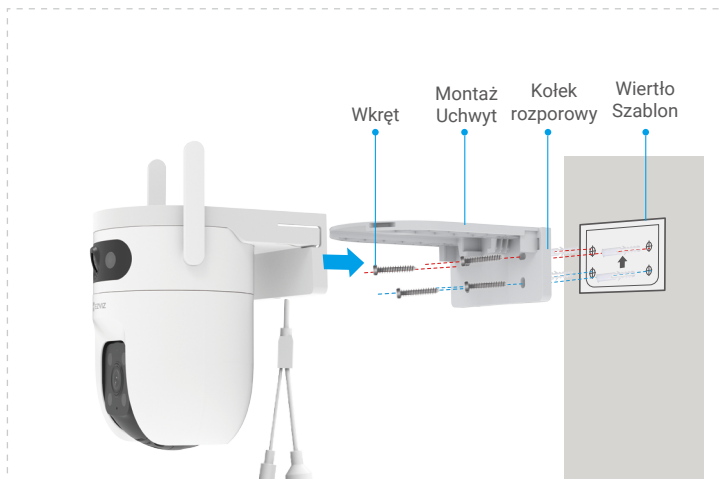
Rys. 2 Montaż ścienny
